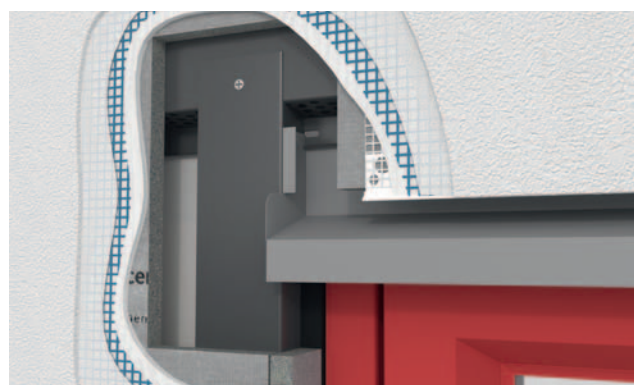
Примыкание надоконного слива
