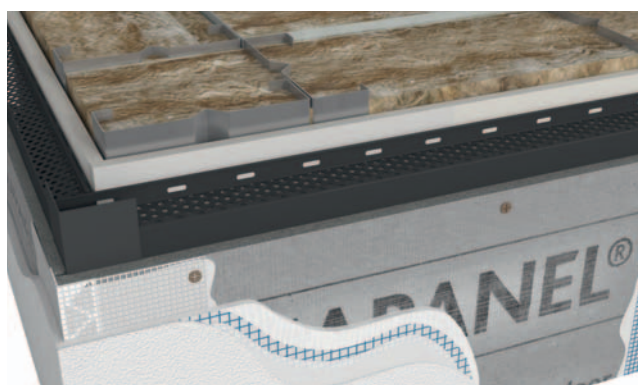
Наружный угол
