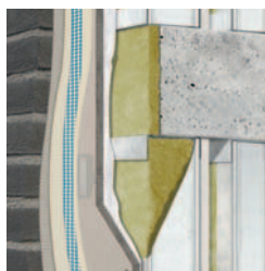
Межэтажное заполнение
