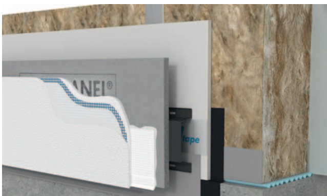
Узел опирания на фундамент
