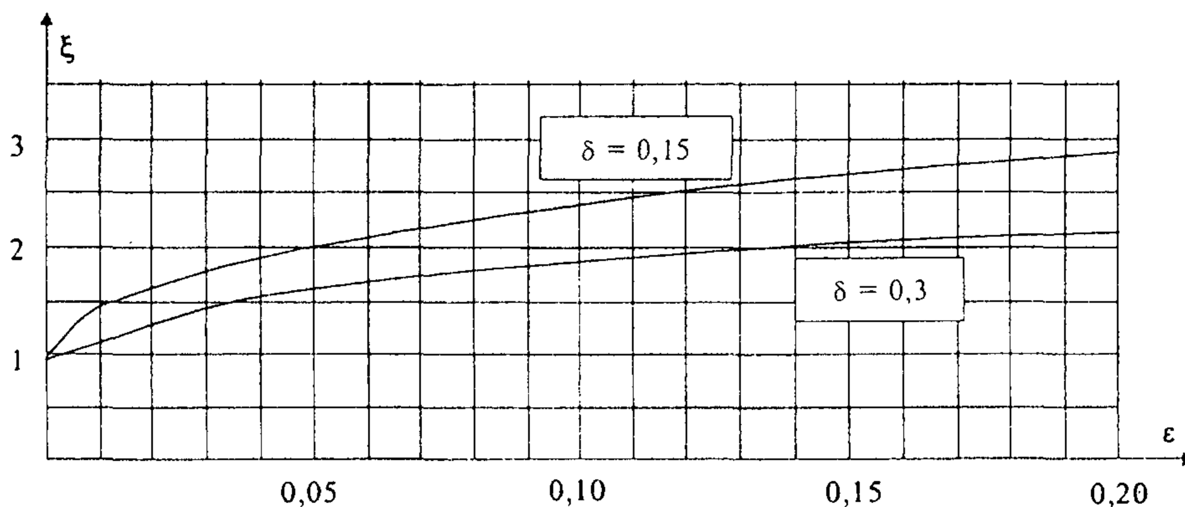
Рисунок 11.1 – Коэффициенты динамичности
